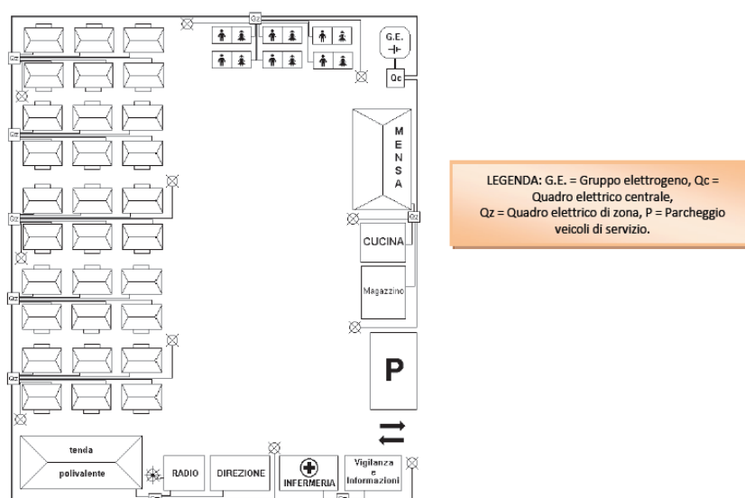
Figura 22: Schema di campo tendopoli su una superficie tipo (dimensioni 100 m x 70 m)
